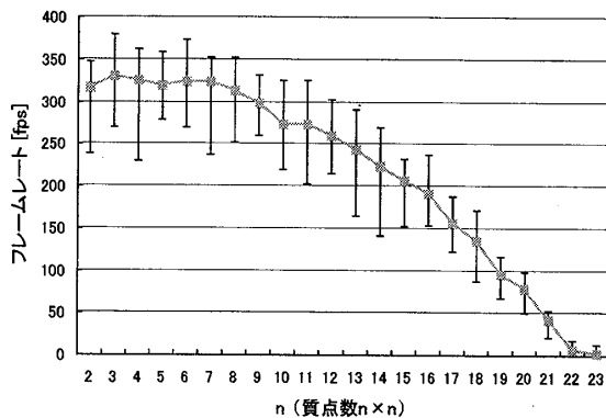
図3 質点数に対するフレームレートの変化
