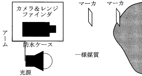
図1：水中遺産計測用カメラモデル
