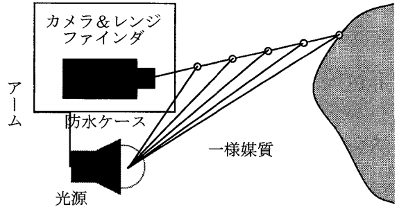
図2：媒質による光の一次散乱モデル ただし、対象表面上の点 \mathbf{r}(z_{surface}) では、媒質ではなく反射角 \theta の拡散反射による減衰が生じるため、以下の式で表される。
