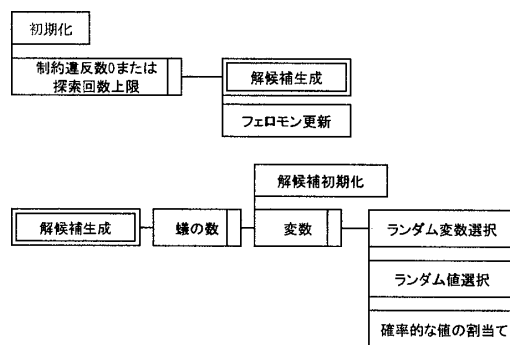
図1 AS のアルゴリズム
