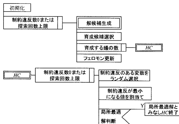
図2 本手法のアルゴリズム
