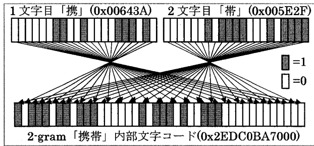
図1 2-gram「携帯」の内部文字コード
