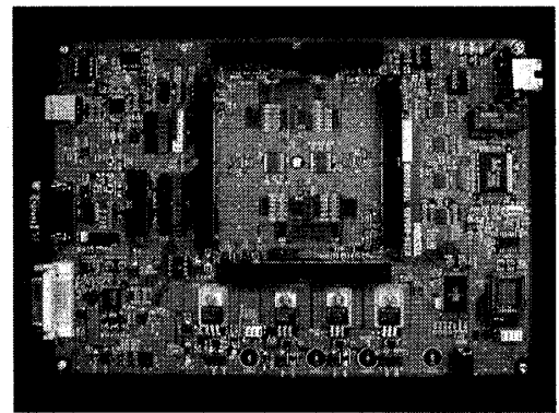
図 2 本研究用に開発した FPGA ボード
