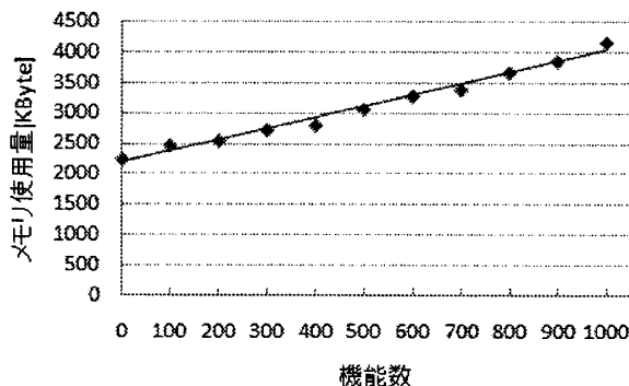
図5 機能数とメモリ使用量の関係
