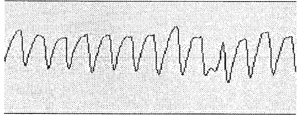
図7. 赤外センサによる脈拍データ 静止状態
