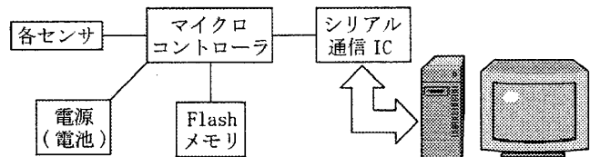
図1. 携帯端末の構成図
