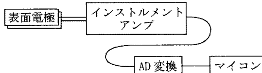
図3. 筋電位測定の流れ
