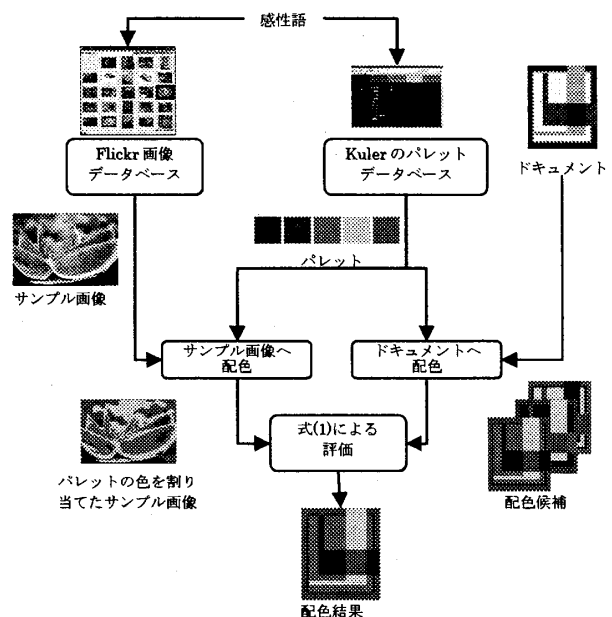
図1 配色処理の流れ
