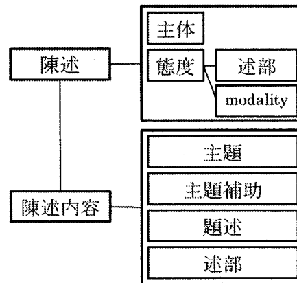
図1: 文構造
