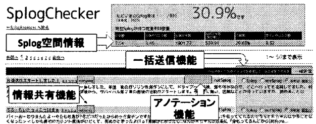
図 3: SplogChecker ユーザインタフェース
