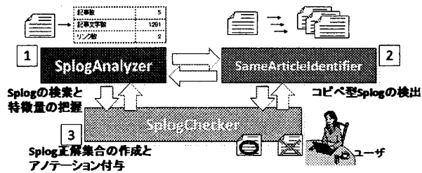
図 1: SplogExplorer 全体構成図
