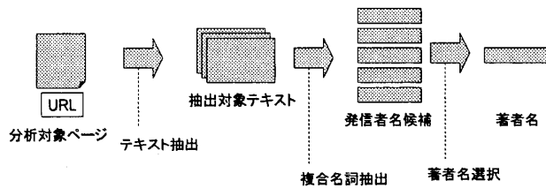
図2: Web ページの著者同定処理の流れ
