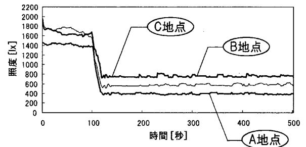
図 4: 照度履歴
