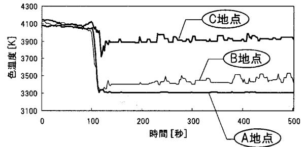
図 5: 色温度履歴
