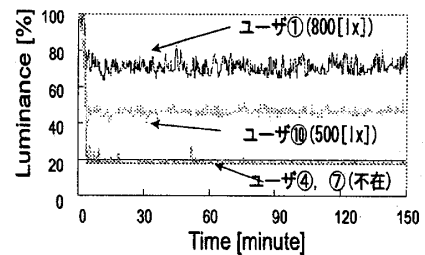
図 6: 光度履歴
