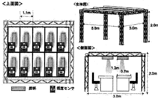
図 2: 構築概要図
