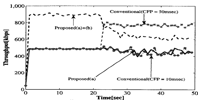
図7: ダウンリンクフロー流量比較
