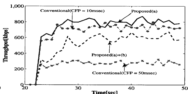
図8: アップリンクフロー流量比較
