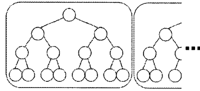
図3: 類似度木
