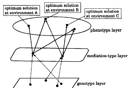
図2 提案手法のモデル図
