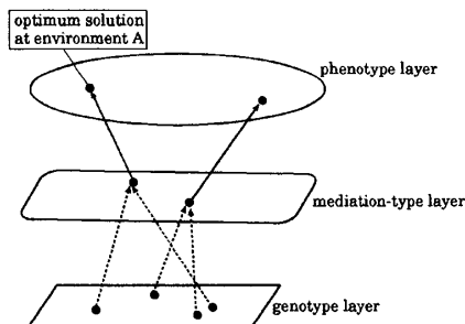
図1 二倍体 GA のモデル図
