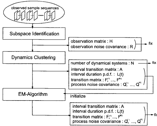
図 2: Hybrid Dynamical System の学習ステップ
