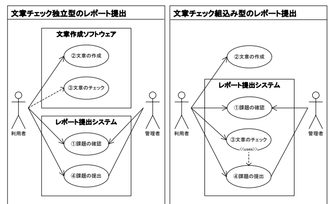
図 5 レポート提出のユースケース図 (右: 提案)
