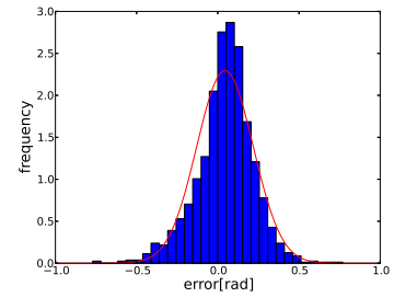
図 3 進行方向推定の誤差分布
