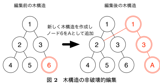
図 2 木構造の非破壊的編集
