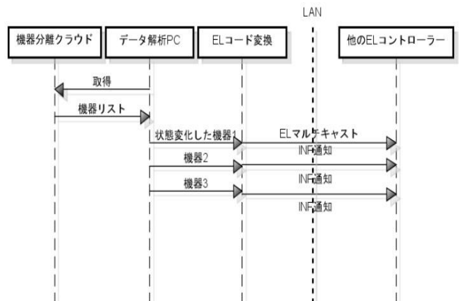
図 5 CloudEL の動作
