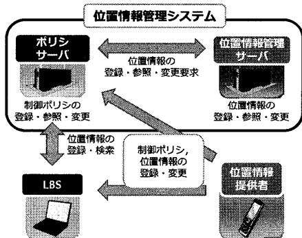
図 3 提案システムの基本構成
