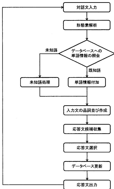
図 2: 対話応答システムの流れ
