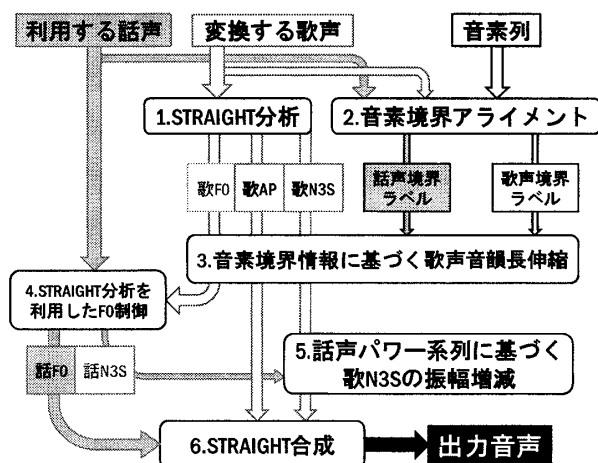
図 2: SpeakBySinging のブロックダイアグラム、F0 は F0 軌跡、AP は非周期性指標系列、N3S はスペクトル系列を表す。図中白抜き箱・点線で示した特徴量・矢印は、音響特徴の制御時のみに使用し、合成時には用いない特徴量を表す。
