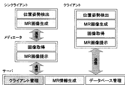
図 2 機能配置図
