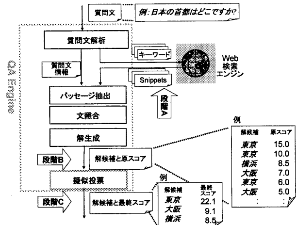
図 1: 基本となる WebQA システム
