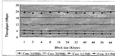
図 4: スループット (1/8)
