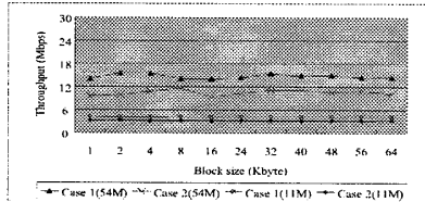
図 3: スループット (1/2)
