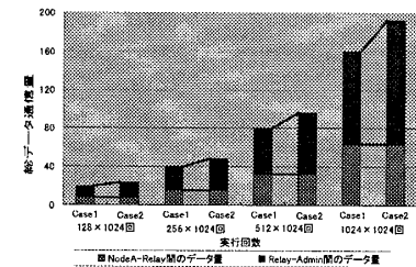
図 6: 総通信データ量
