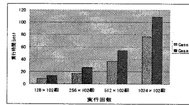
図 5: 実行時間
