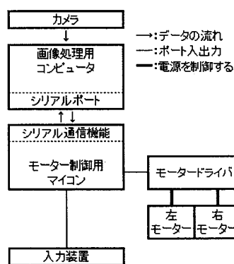
図 2 制御装置間の接続図
