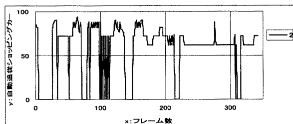
図5 自動追従ショッピングカートの速度
