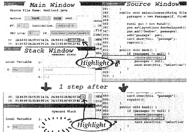
図 1: 逐次実行による画面変化
