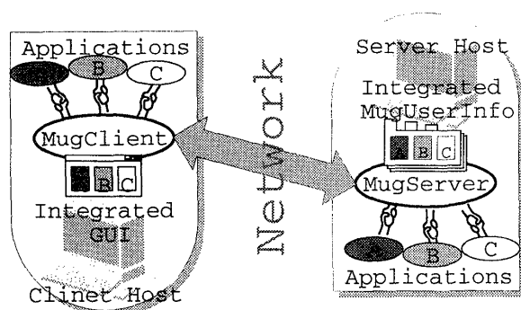
図 1: マルチユーザ・フレームワーク Mug
