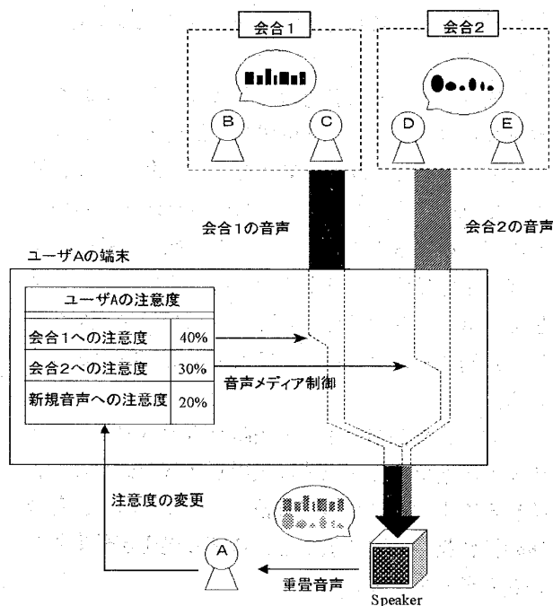
図2 注意度に応じた音声メディア制御
