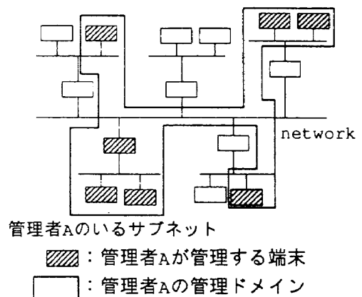
図 1: PICKLES 端末群の管理ドメイン
