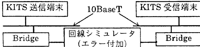
図2 実験ネットワーク構成
