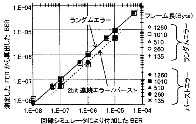
図3 設定したBERとFERから算出したBERの関係
