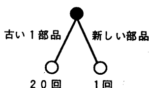
図2 推定木の例
