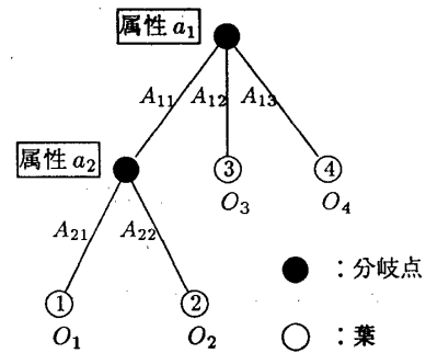
図 1 推定木
