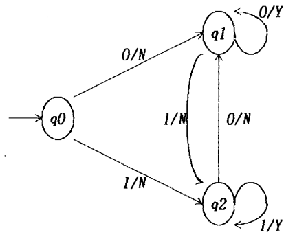
図 5. 推測された Mealy 型オートマトン
