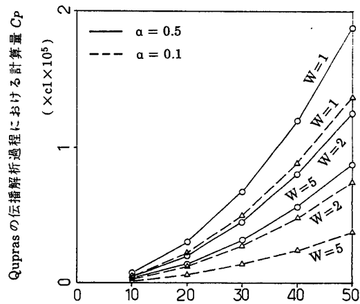
各クラス・オブジェクトに含まれるインスタンスの個数 K <方法1による W 等分分割モデルの各パラメータ値> S=50, c_1=c_2, R'=1, K=10 \rightarrow 50, W=1 \rightarrow 5, \alpha=0.1 \rightarrow 0.5
