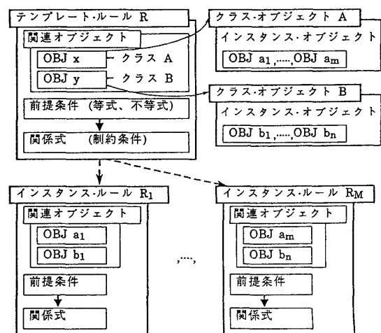
図1. Quprasの知識表現とインスタンス・ルールの生成
