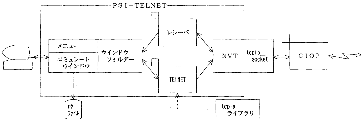
図2 PSI-TELNETの構成
