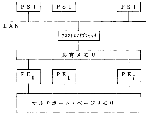
図1 Mu-Xのハードウェア構成
