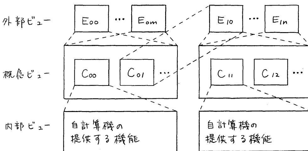
図1 SBSの三層ビュー
