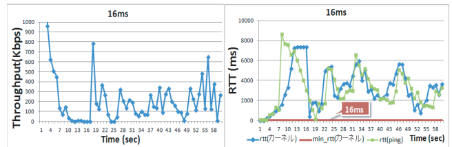
図5: スループットと往復遅延時間の遷移
