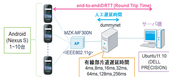
図 2: 実験トポロジ
