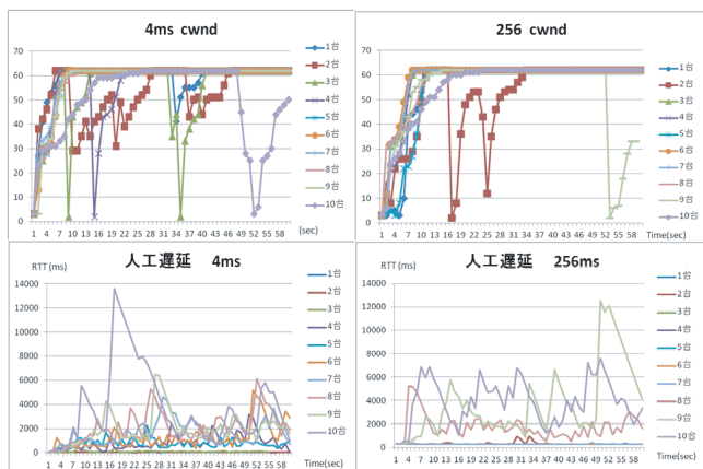
図4: 輻輳ウィンドウと実際の遅延時間の遷移
