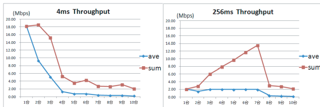
図3: 通信台数の変化によるスループットの平均値, 合計値
