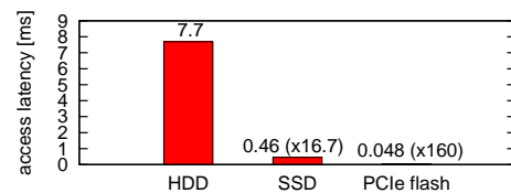
図 2: 16KB ランダム読み込みのアクセス遅延と、HDD に対する性能比
