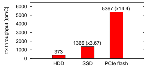
図 4: TPC-C のトランザクションスループットと、HDD に対する性能比
