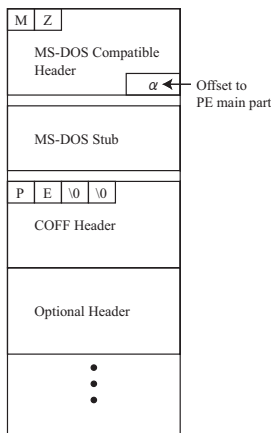
図 7 PE 形式の構造
