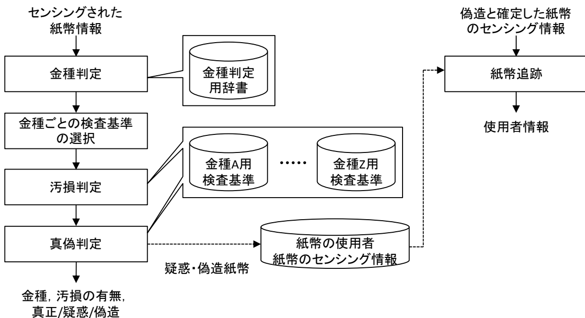
図2 紙幣識別の流れ
