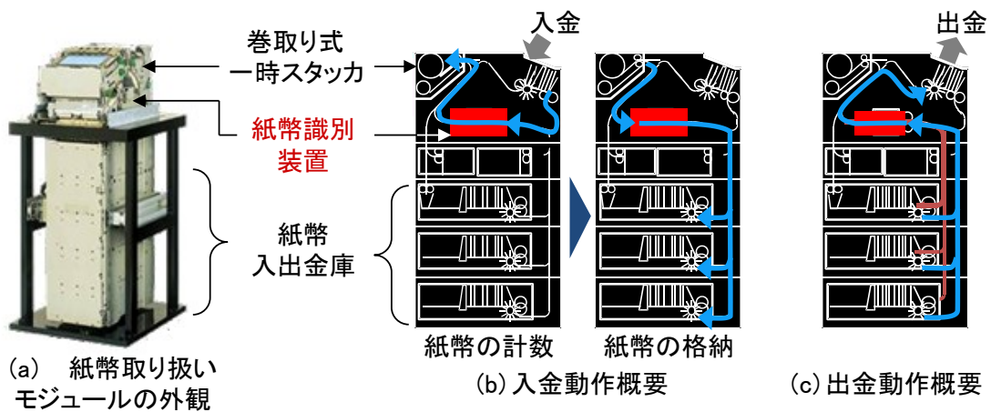
図1 紙幣識別モジュールと入金/出金動作
