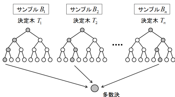
図 3 ランダムフォレスト
