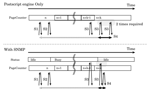
図 4 総印刷枚数取得までのタイムダイアグラム
