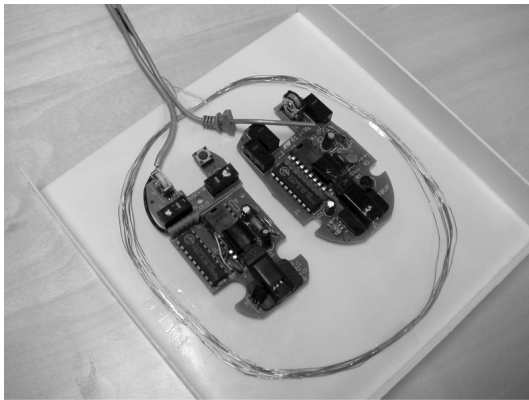
図 1 MouseField 装置の実装例。2 個の光学マウスユニットの周囲に、RFID リーダのアンテナを配置
