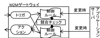
図4：ルールベース自律分散機器制御
