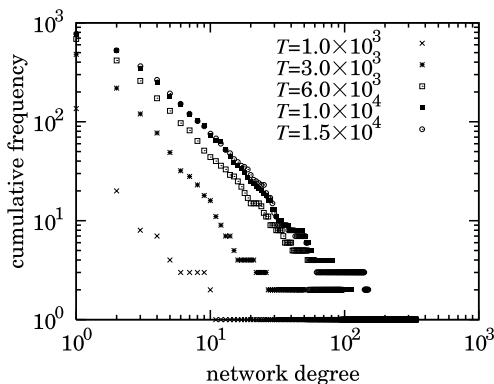
図 8 次数分布の時間発展
