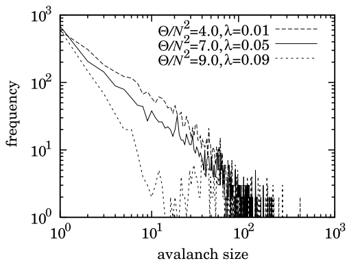
図 5 進化の雪崩のサイズの分布
