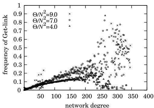
図 6 各次数のノードごとのリンク追加頻度
