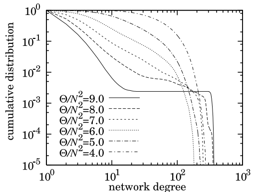
図 1 次数分布 Fig. 1 Degree distribution.
