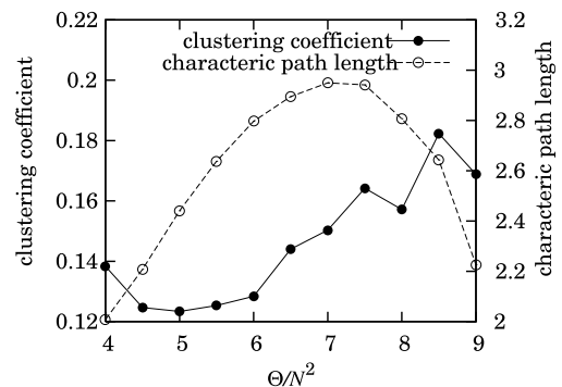
図3 クラスタリング係数，平均経路長 Fig.3 Clustering coefficient and characteristic path length.
