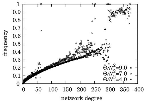
図 7 次数に対するリセット頻度
