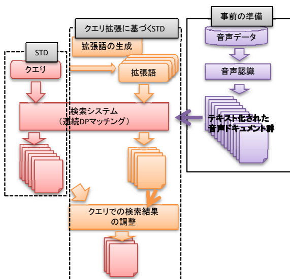
図 1 クエリ拡張に基づく STD の概要
