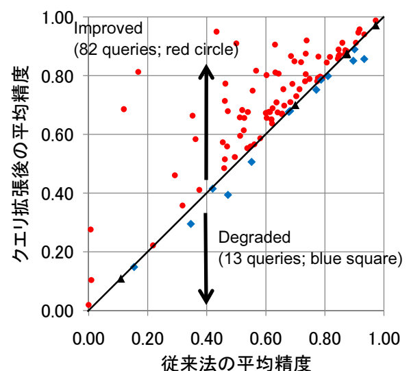
図 2 文字列を付加するクエリ拡張の効果 (クエリごとの分析) 拡張: 前後の併用, penalty=2.5
