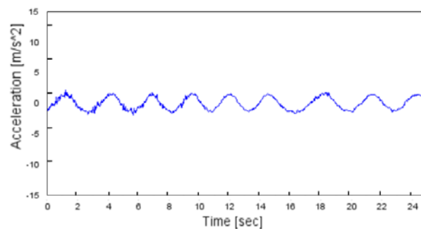
図 4 ICA により分離された信号(1)
